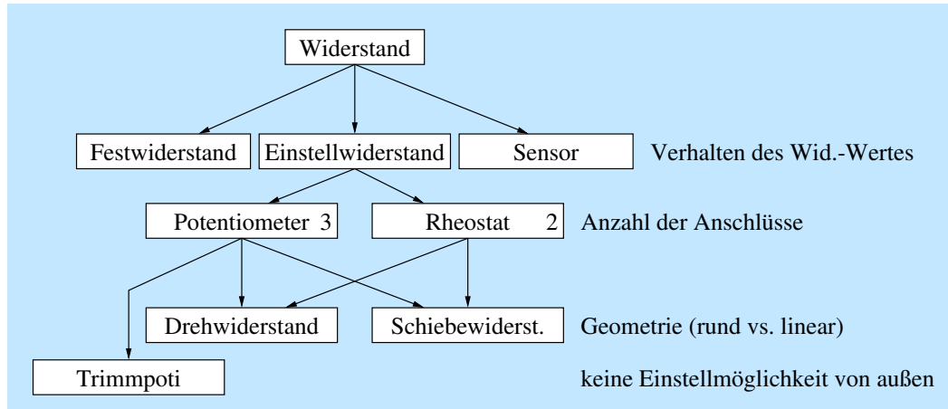
Abbildung 1: Arten technischer Widerstände
